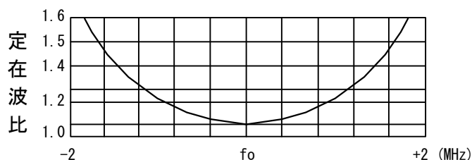
周波数特性
