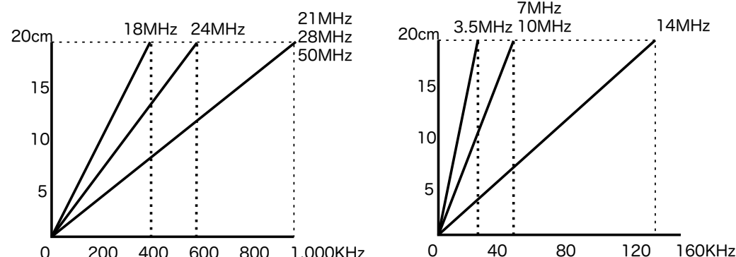
エレメント折曲げによる周波数変動
