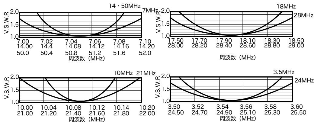
周波数特性
